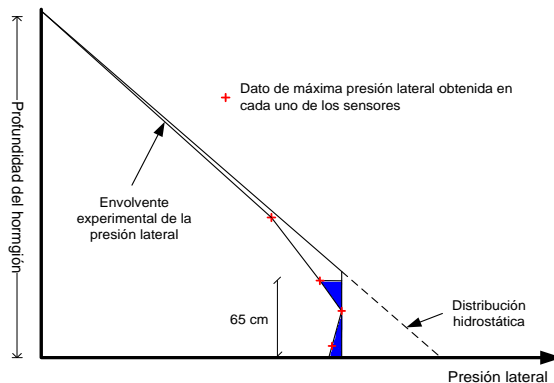
Figura III.- Grafica de comparación entre la envolvente de presión real y una distribución bilineal para el mismo valor de máxima presión lateral
